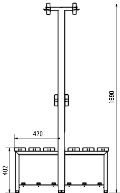
Wymiary ławko-wieszaka dwustronnego podane w mm
